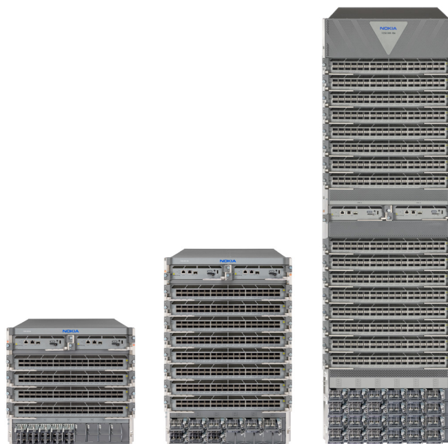
7250 IXR-6e
